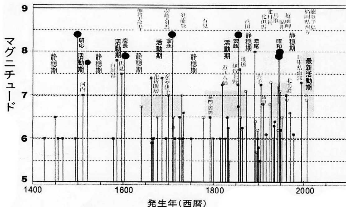
図 3. 南海トラフの巨大地震と内陸直下地震
